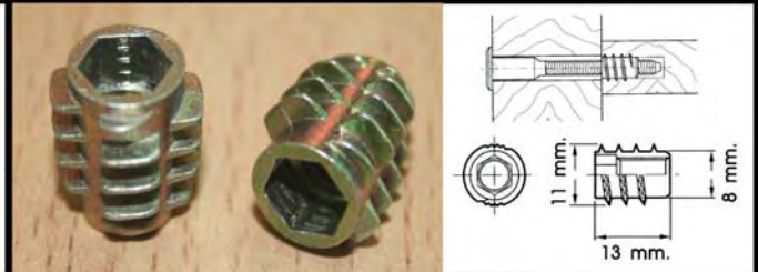
DRIVING NUT E-TYPE / น๊อตฝังไม้แบบไม่มีบ่า
