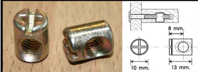
CROSS DOWEL / เดี่ยวขวาง
