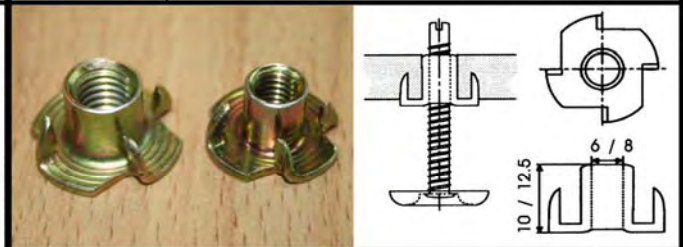
T-NUT / ดาวกระจาย
