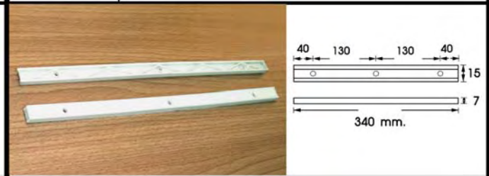
PLASTIC DRAWER SLIDE / รางลิ้นชักพลาสติก
