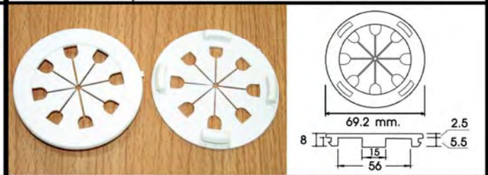
PLASTIC WIRE CAP FOR BACK CABINET / ฝาร้อยสายไฟหลังตู้
