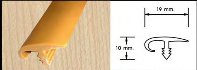
PLASTIC PROFILE FOR FURNITURE / คิ้วปิดขอบเฟอร์นิเจอร์
