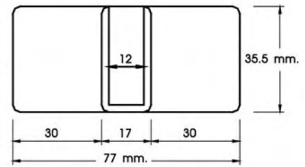
PLASTIC CONNECTING JOINT FOR THICKNESS BOARD 12 MM. / ตัวประกอบเฟอร์นิเจอร์ สำหรับไม้หนา 12 มม.
