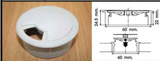
PLASTIC WIRE CAP / ฝาร้อยสายไฟ
