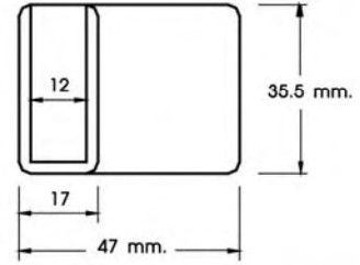
PLASTIC CONNECTING JOINT FOR THICKNESS BOARD 12 MM. / ตัวประกอบเฟอร์นิเจอร์ สำหรับไม้หนา 12 มม.
