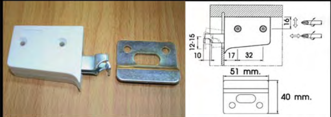
BRACKET WITH STEEL PLATE / ตัวแขวนตู้พร้อมแป้นรองรับ
