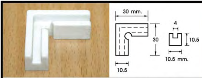
PLASTIC CONNECTING JOINT / ตัวยึดมุมเฟรมอลูมิเนียม
