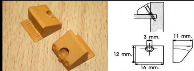
PLASTIC BACK PANEL FITTING / ตัวยึดหลังตู้
