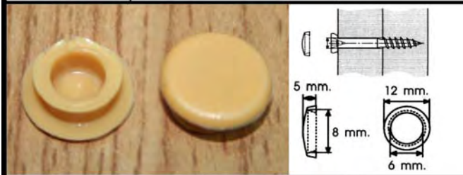
PLASTIC COVER CAP / ฝาปิดรูน็อต แบบมีบัว
