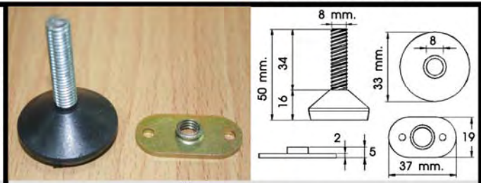
ADJUSTABLE LEG / น๊อตขาปรับระดับ
