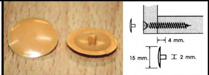
PLASTIC COVER CAP / ฝาปิดรูน็อต แบบแกนสั้น
