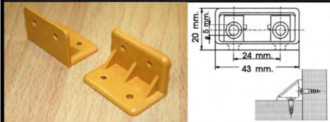
PLASTIC CONNECTOR L SHAPE / ฉากลิ้นชักตัวใหญ่รูปแบบ L
