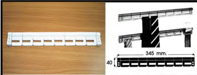
PLASTIC NECKTIE RACK / รวแขวนเนคไท
