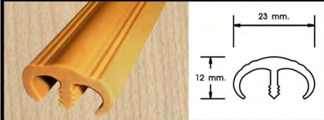
PLASTIC PROFILE FOR FURNITURE / คิ้วปิดขอบเฟอร์นิเจอร์
