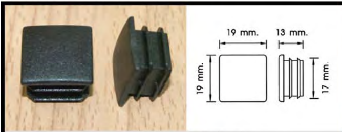
PLASTIC END CAP TUBE / ฝาปิดท่อสี่เหลี่ยม
