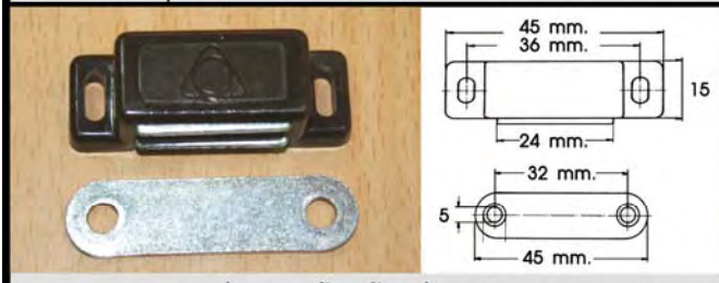
MAGNETIC / แม่เหล็กพร้อมลิ้นแผ่นเหล็กแบบ 1 รูและ 2 รู
