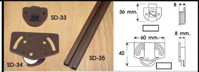
SLIDE DOOR SYSTEM / ลูกล้อปรับระดับได้
