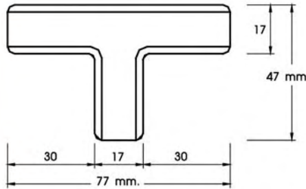
PLASTIC CONNECTING JOINT FOR THICKNESS BOARD 12 MM. / ตัวประกอบเฟอร์นิเจอร์ สำหรับไม้หนา 12 มม.
