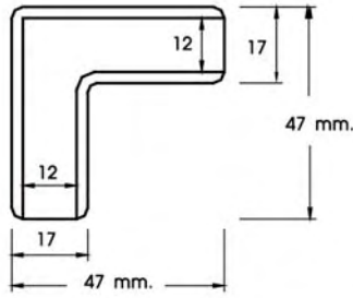
PLASTIC CONNECTING JOINT FOR THICKNESS BOARD 12 MM. / ตัวประกอบเฟอร์นิเจอร์ สำหรับไม้หนา 12 มม.
