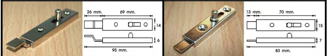
BENDED STEEL BOLT / กลอนประตู่ข้าง
