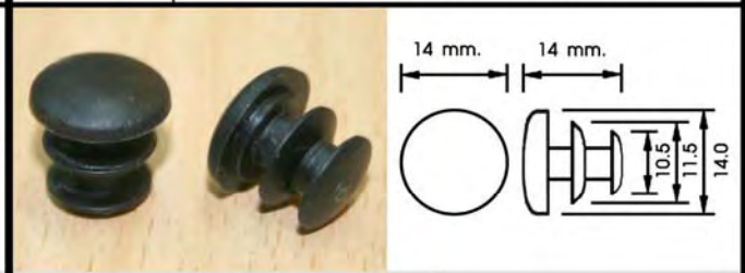
PLASTIC END CAP TUBE / ฝาปิดทอกลม
