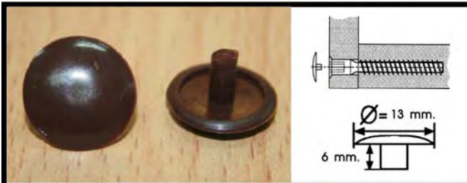
PLASTIC COVER CAP / ฝาปิด CFM แกนยาว
