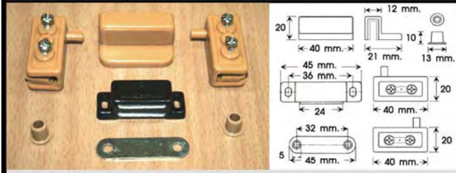
PLASTIC GLASS HINGES / ตัวหนีบกระจกมือจับแม่เหล็ก
