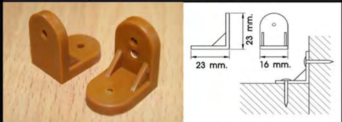
PLASTIC CONNECTOR L SHAPE / ฉากลิ้นชักตัวเล็กรูปแบบ L
