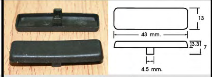
PLASTIC HINGE'S CAP / ฝาปิดบานพับ
