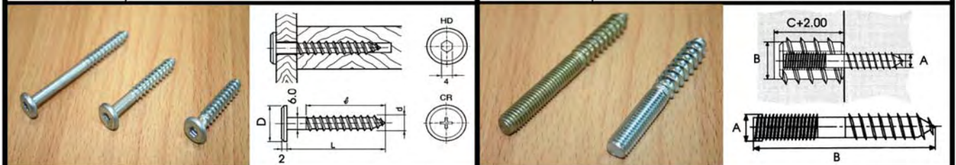
CHIPBOARD SCREWS / สกรูหกเหลี่ยม JCB เกลียวปล่อย
