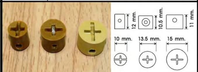
PLASTIC CROSS DOWEL / น๊อคดาวน์
