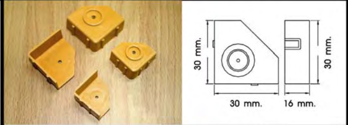
PLASTIC CORNER V SHAPE / กันกระแทกรูปตัว V
