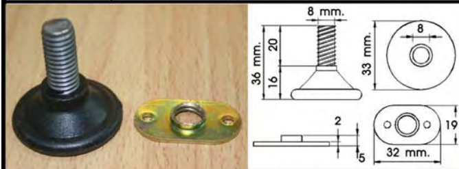
ADJUSTABLE LEG / น๊อตขาปรับระดับ
