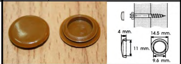
PLASTIC COVER CAP / ฝาปิดรูน็อต แบบมีบัว
