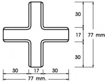
PLASTIC CONNECTING JOINT FOR THICKNESS BOARD 12 MM. / ตัวประกอบเฟอร์นิเจอร์ สำหรับไม้หนา 12 มม.
