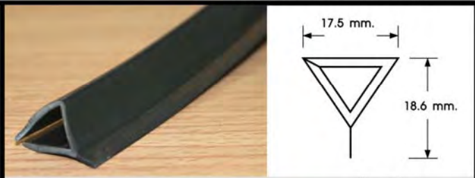
PLASTIC WATERPROOF PROFILE / ยางรองขาตู้กันน้ำซึม
