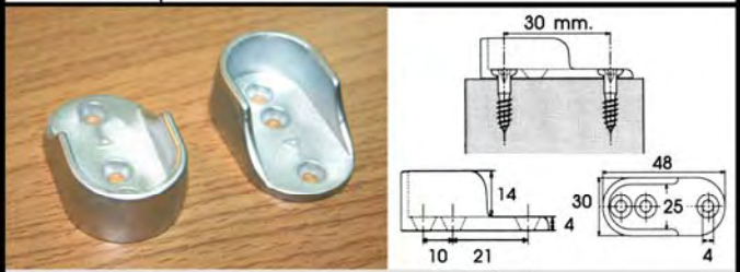
PLASTIC TUBE HANGER / ตัวแขวนราวเสื้อผ้าพลาสติก
