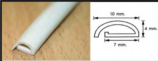
PLASTIC BUMPER PROFILE / ยางกันกระแทกพลาสติก
