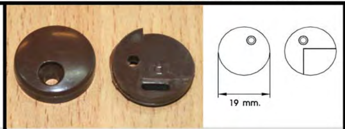
PLASTIC MIRROR FITTING / มุมยึดกระจก
