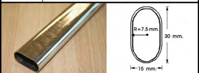
METAL TUBE (STEEL, STAINLESS) / รวแขวนแบบวงรี
